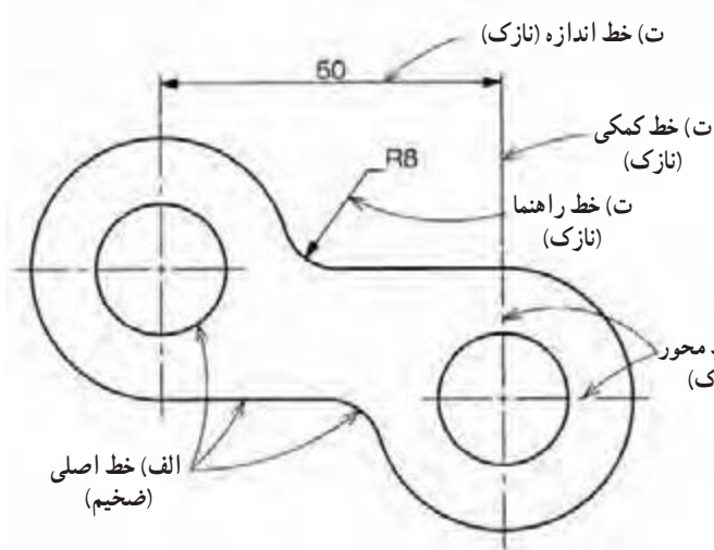
شکل ۱۹-۸. حالات مختلف کاربرد خط
