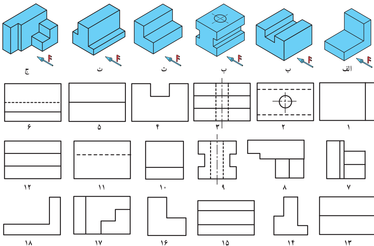
شکل ۸-۲۶. تصاویرهای سه بعدی قطعه‌ها به همراه نماهای آن‌ها
